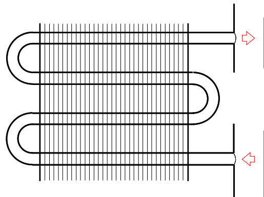
Principle of Liquid Circuit Prinzip die Flüssigkeitkreislauf Princippet i Væskekredsløb
